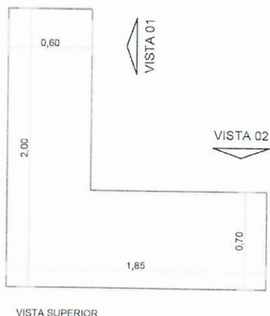
VISTA SUPERIOR
