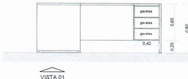
VISTA 01
