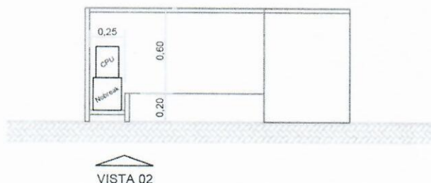
VISTA 02
