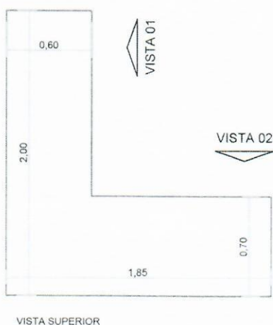
VISTA SUPERIOR
