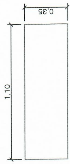
PLANTA BAIXA ARMÁRIO AÉREO EM MADEIRA VISTA 01
